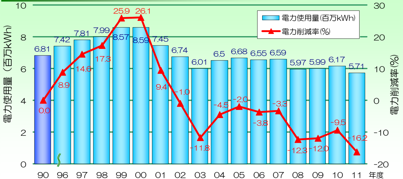
群馬工場 空調設備入替え
